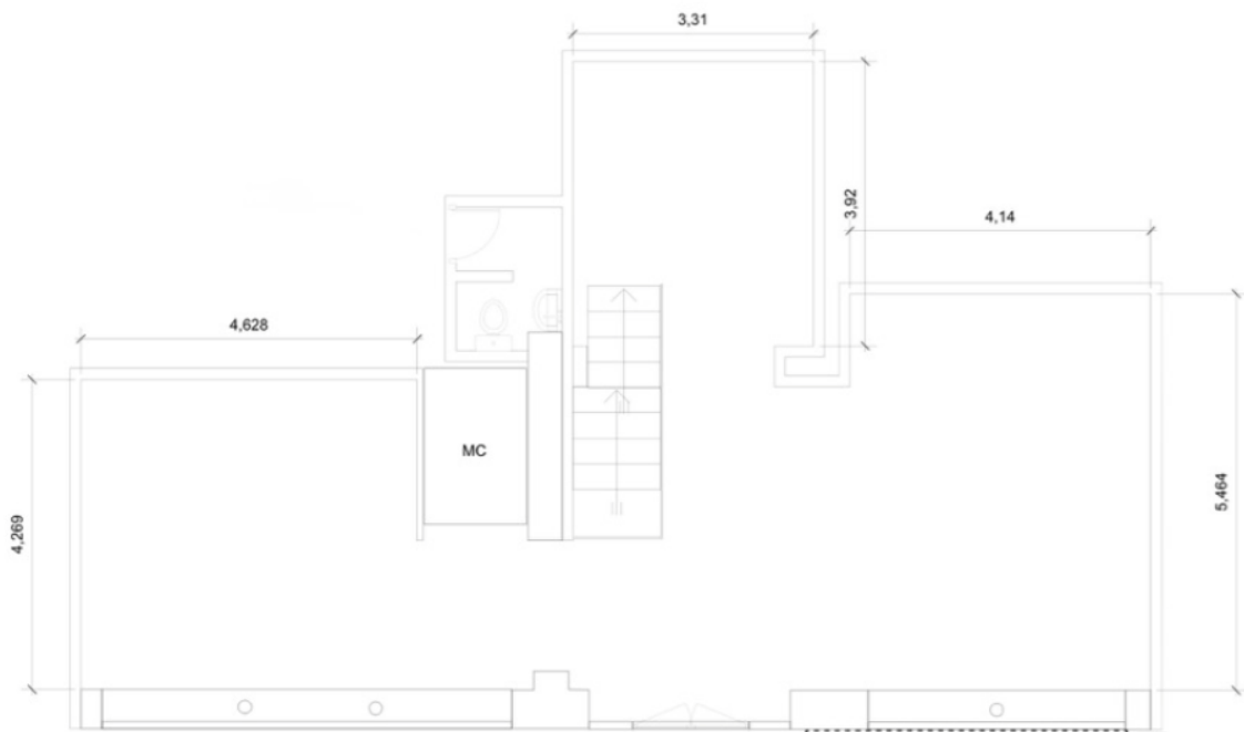
Plan rez-de-chaussée, 90 m2
